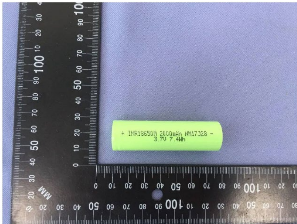
Abb.1 Gesamtansicht I des Akkus
